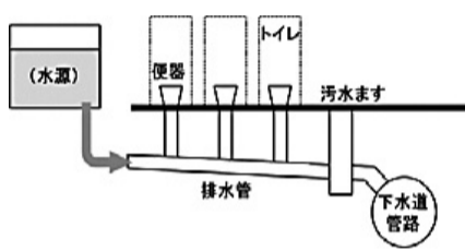
貯留型マンホールトイレの模式図。下水道管につながるように接続し、プールの水などを水源に流せるようになっています。[けんせつ Plaza] ホームページより (http://www.kensetsu-plaza.com/kiji/post/18770)
