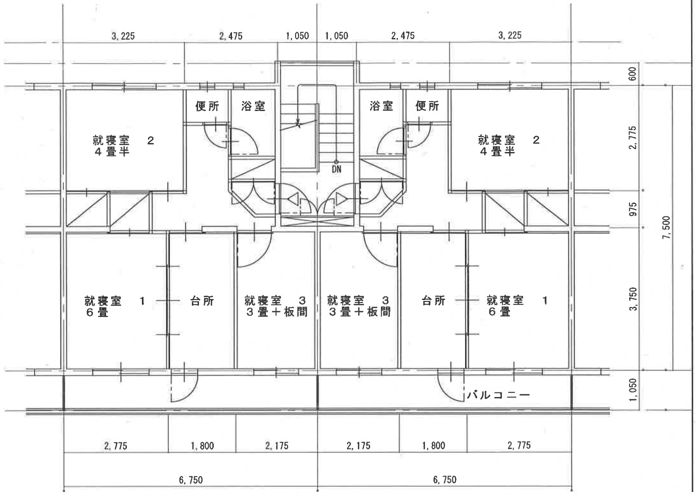
1 ~ 4 階 間 取 図 (A 棟、B 棟 共 通) S=1:100
